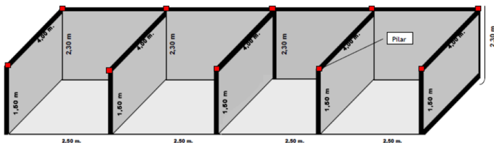
Figura 29: Exemplo de modelo de estrutura com baias de alvenaria.
