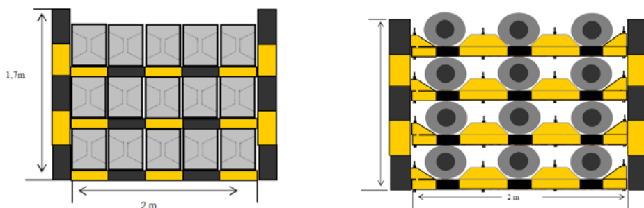
Figura 19: Armazenagem de poste (duplo T) armazenamento de poste (Circular).
